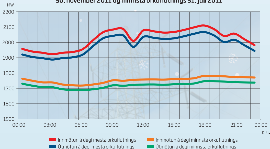
Dægursveifla á afli innmötunar og úttektar á degi mesta orkuflutnings 30. nóvember 2011 og minnsta orkuflutnings 31. júlí 2011
