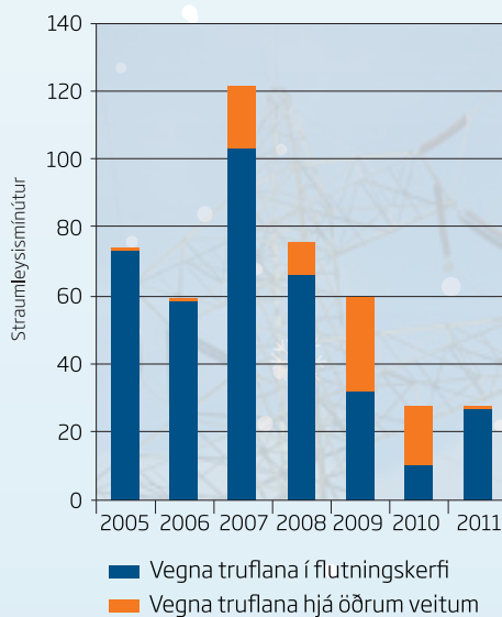
Straumleysismínútur vegna fyrirvaralausra rekstrartruflana
